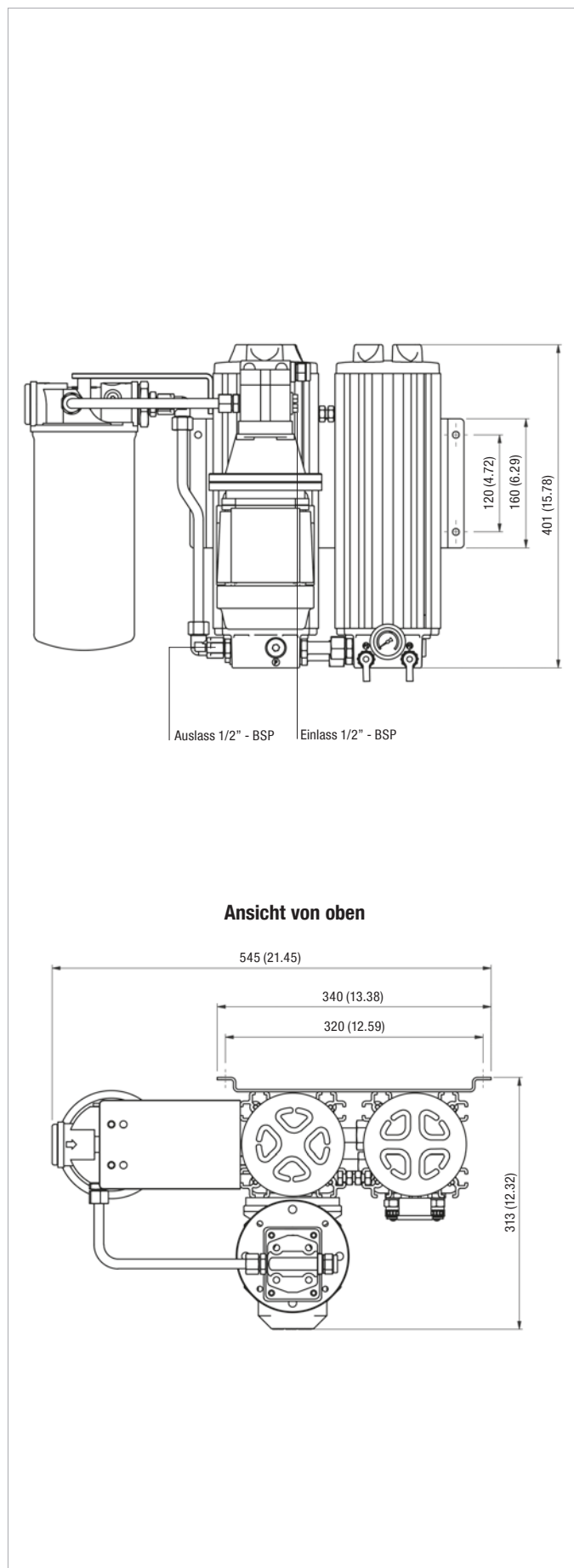
Abmessungen OLSW-2-30
