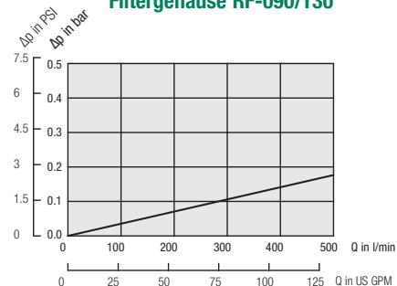
Filtergehäuse RF-090/130
