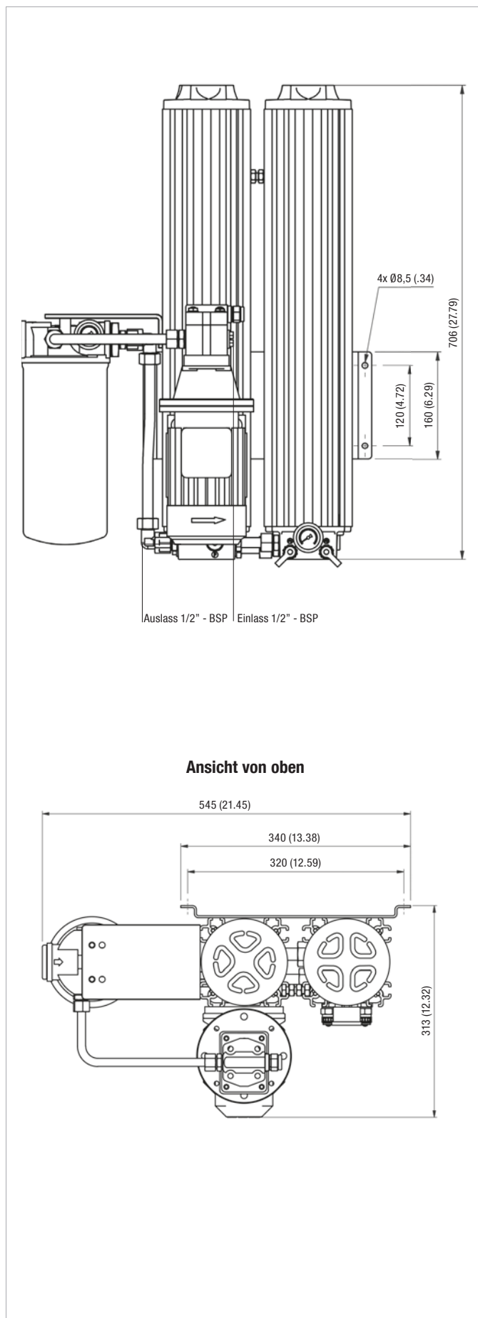
Abmessungen OLSW-2-60
