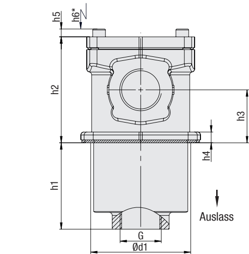
RFS-045/070
