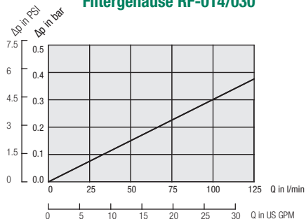
Filtergehäuse RF-014/030
