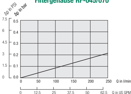
Filtergehäuse RF-045/070
