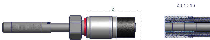
Bild 4: Minimaler Nippeleinfall
