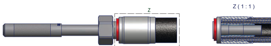
Bild 3: Optimaler Nippel einfall
