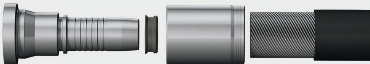
Standard ECOVOS Schlauchnippel
