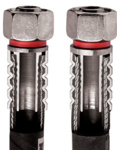
Non-Skive (für Nicht-Schälung)
